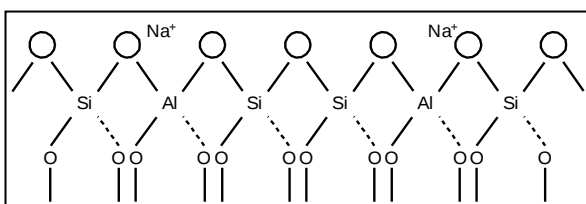
Gambar 2.2. Struktur Sisi Aktif Dalam Zeolit
