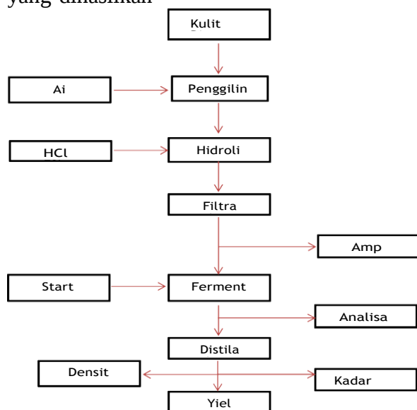
Gambar 2. Skema Proses Pembuatan Bioetanol dari Kulit Pisang Kepok
