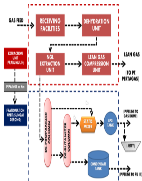
Gambar 2.1. Skema Proses Pembuatan LPG Kilang PT Perta-Samtan Gas
