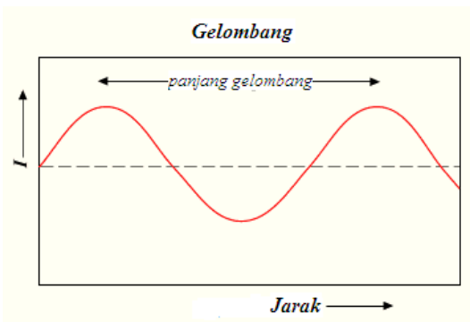
Gambar 1.1 Panjang Gelombang
