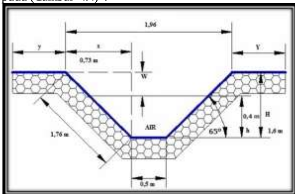
Gambar 4.4 Bentuk Saluran Tambang Aktual
