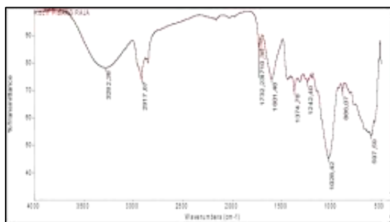
Gambar 4.1 Analisa FTIR
