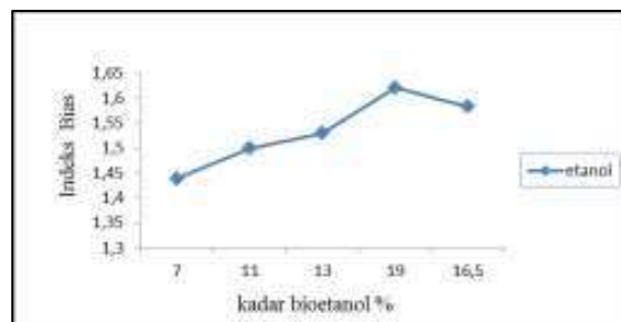
Gambar 4.3 Grafik Hubungan Indeks Bias Terhadap Kadar Bioethanol
