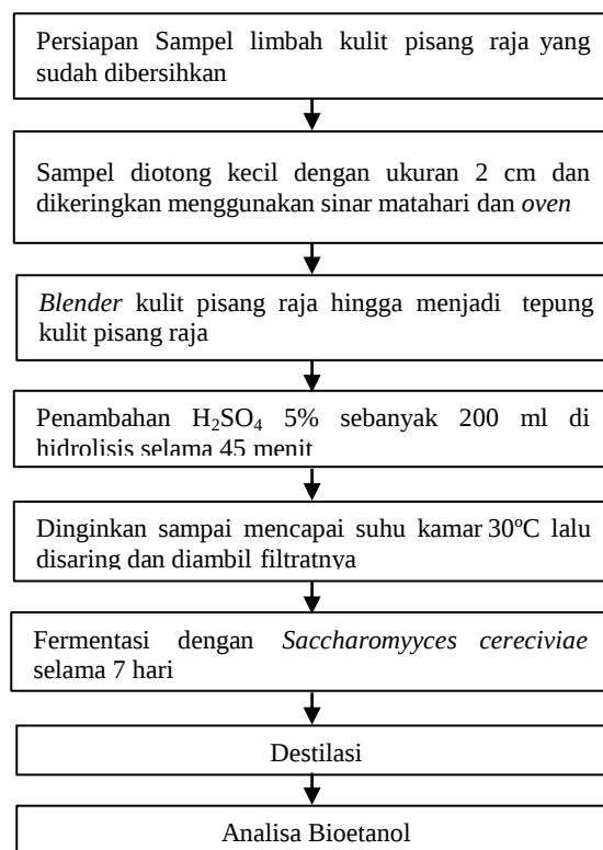
Gambar 3.1 Diagram Alir Proses Pembuatan Bioetanol
