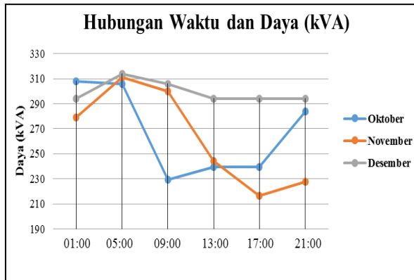
Gambar 4.2 Grafik Hubungan Waktu dan Daya
