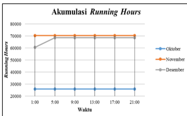
Gambar 4.3 Grafik Akumulasi Running Hours
