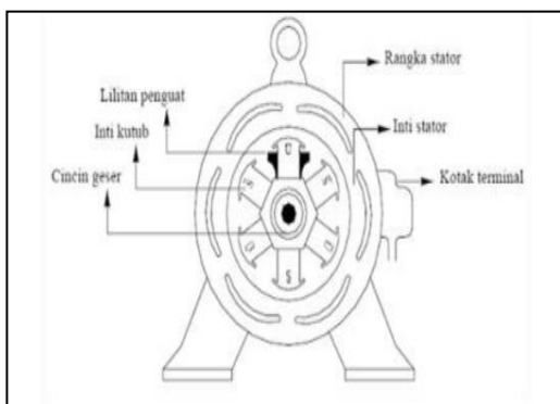
Gambar 2.2 Kontruksi Generator Sinkron
