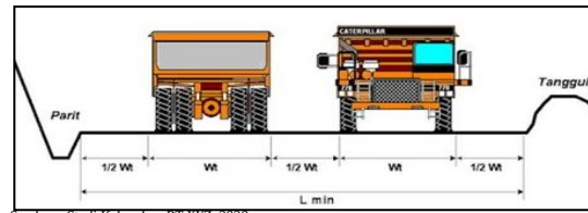
Gambar 3.4 Dimensi Jalan Tambang
