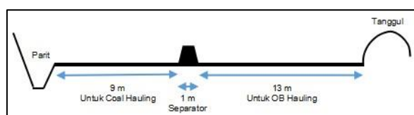
Gambar 3.9 Pembagian Jalan
