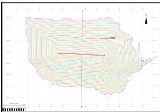
Gambar 3.5 Desain Pit dan Jalan Angkut Pit Alam 1-3 dengan 1 Akses Jalan
