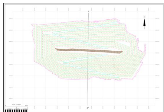
Gambar 3.7 Desain Pit dan Jalan Angkut Pit Alam 1-3 dengan 2 Akses Jalan
