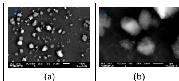
Gambar 4.4 Hasil Pengujian SEM sampel toner 15 CB dengan perbesaran: (a) 1000 dan (b) 8000 kali
