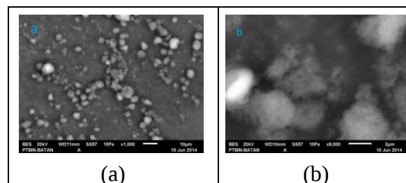
Gambar 4.3 Hasil Pengujian SEM Sampel Toner 10 CB dengan perbesaran: (a) 1000 dan (b) 8000 kali
